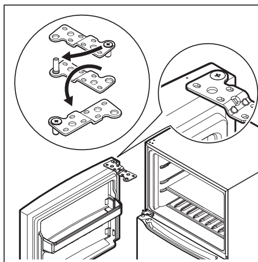
Type B hinge
